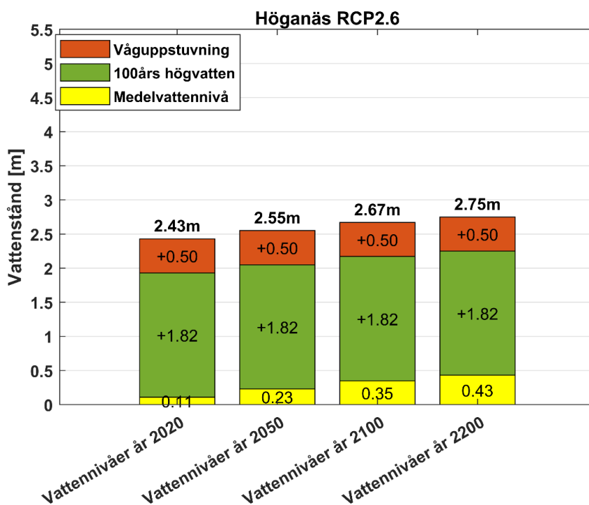
Figur 13 Bidragande komponenter till framtida möjlig vattenståndsökning i Höganäs med klimatscenario RPC2.6 i grunden. Ingående komponenter är medelvattenstånd (gult), 100-års högvatten (grönt) samt våguppstuvning (rött).
