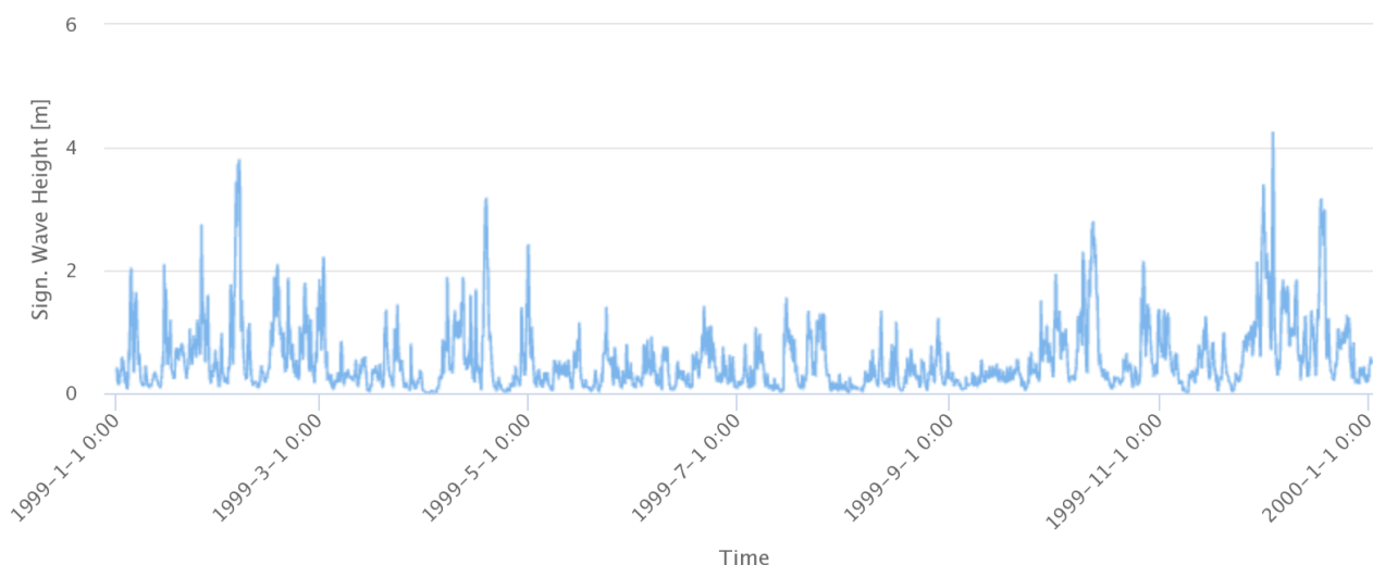
Figur 8 Tidsserie av signifikant våghöjd utanför Höganäs kust på ca 20 m djup.
