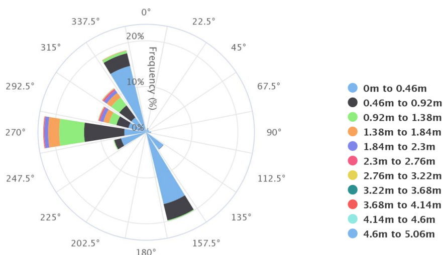
Figur 9 Vågros för signifikant våghöjd utanför Höganäs på ca. 20 m djup. Denna visar hur ofta (andel av tiden) vågorna kommer från en viss riktning. Våghöjden, i varje sektor, anges i en färgskala.
