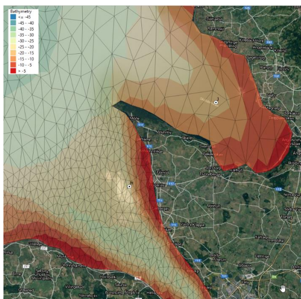
Figur 7 Förstoring av modellens batymetri (djup) och beräkningsnät i området.
