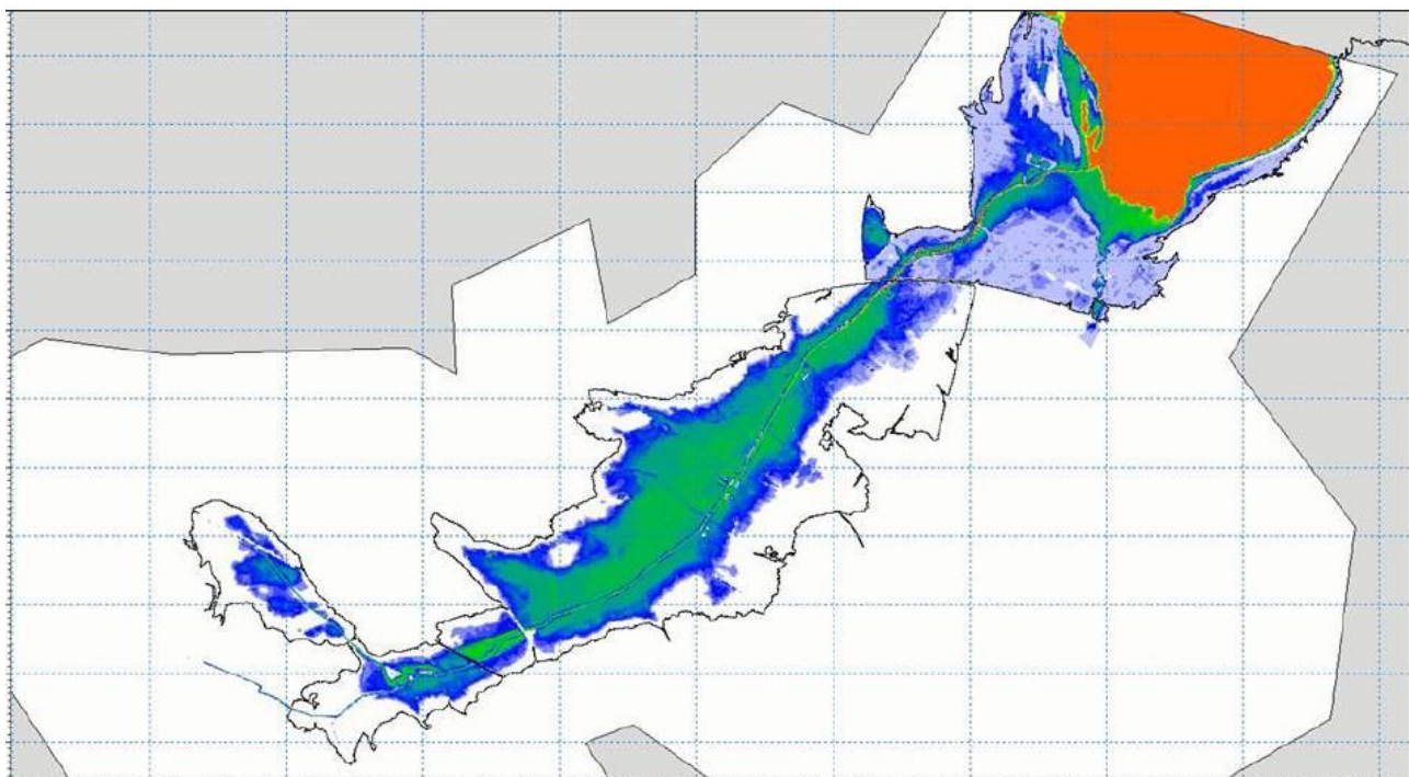
Figur 2 Maximal översvämningsutbredning uppströms väg 112 längs Görslövsån i samband med ett framtida 100-års vattenstånd med varaktighet motsvarande adventsstormen den 27 november 2011. Observera att den maximala utbredningen och vattendjupet nedströms väg 112 inträffar vid en tidigare tidpunkt. (Från DHI, 2013).
