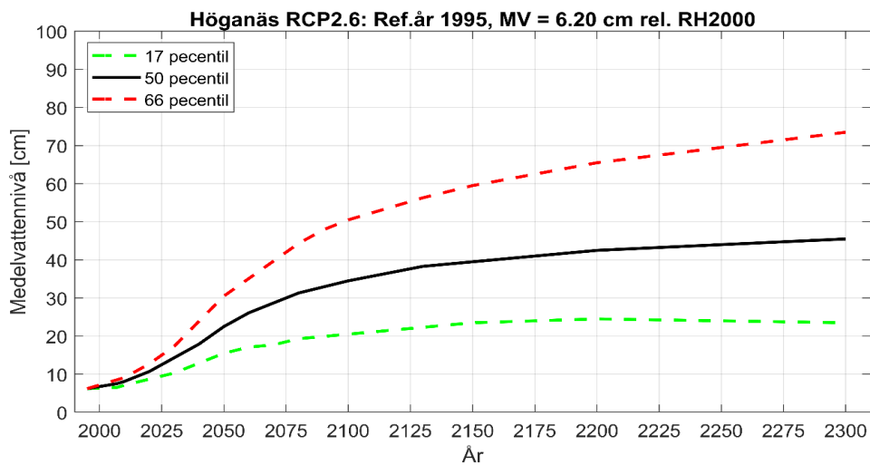
Figur 11 Den framtida medelvattennivån för IPCC scenario RCP2.6 för Höganäs kommun fram till år 2300. Den svarta linjen visar centralestimatet medan med övre (röda streck) och undre (gröna sträck) konfidensintervall.
