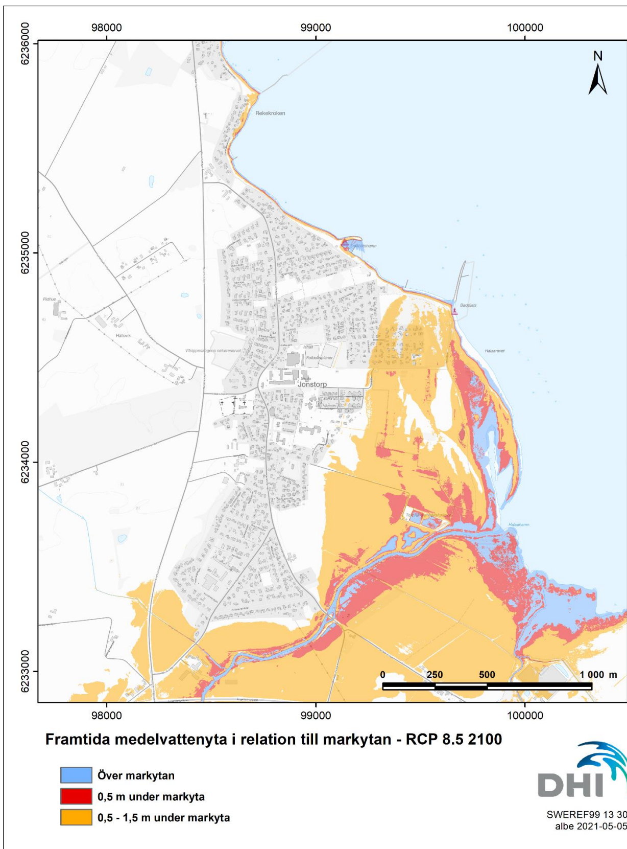
Figur 35 Framtida medelvattenyta i relation till markytan för scenario RCP 8,5 år 2100.
