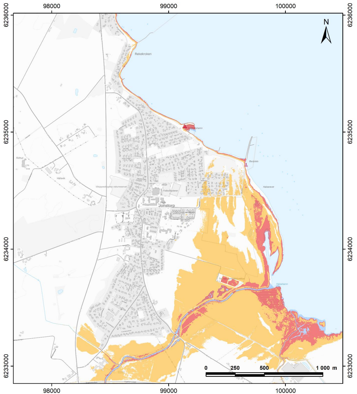
Framtida medelvattenyta i relation till markytan - RCP 2.6 2100
