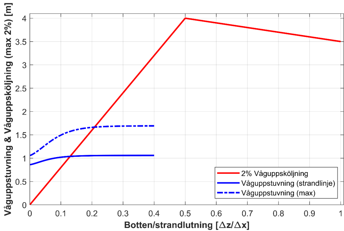
Figur 19 Våguppstuvning (blå heldragen och streckad linje) och våguppspolning (röd linje) för Höganäs för inkommande vågor med signifikant höjd 4m och period 8s.
