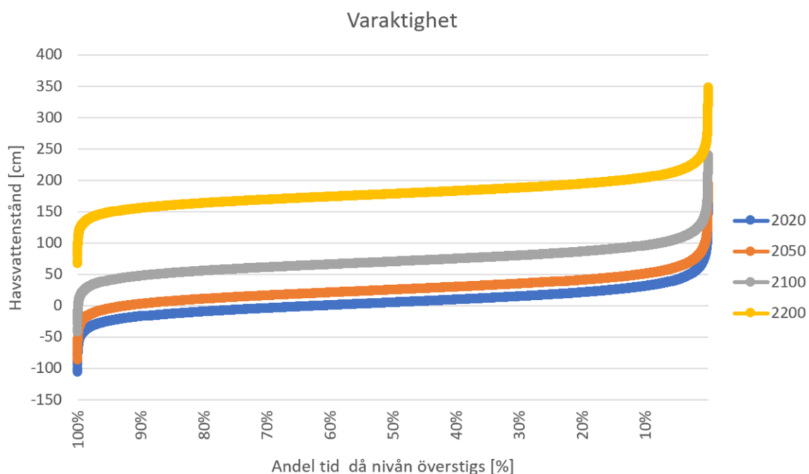
Figur 17. Varaktigheten för vattenstånd vid Viken visas för 2020 (baserat på SMHI's mätdata 1977-2020) samt motsvarande för framtida nivåer (scenario RCP8.5).
