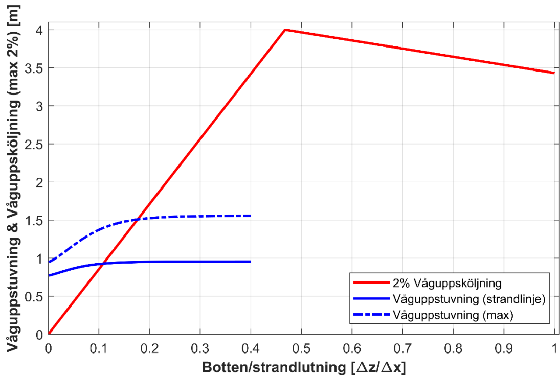
Figur 20 Våguppstuvning (blå heldragen och streckad linje) och våguppspolning (röd linje) för Jonstorp för inkommande vågor med signifikant höjd 3.5m och period 8s.
