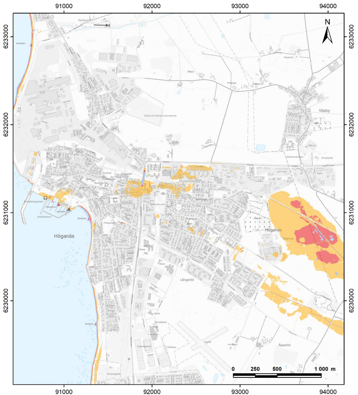
Framtida medelvattenyta i relation till markytan - RCP 8.5 2100
