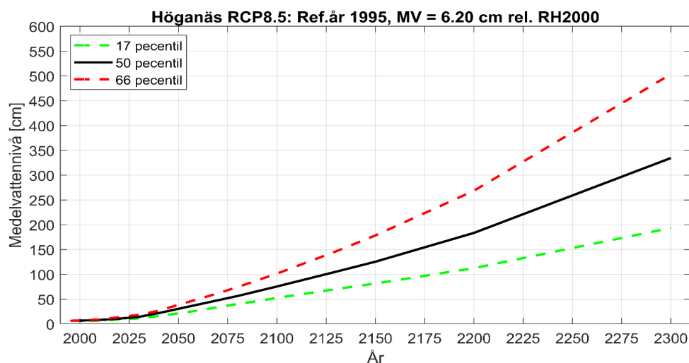
Figur 12 Den framtida medelvattennivån för IPCC scenario RCP8.5 för Höganäs kommun fram till år 2300. Den svarta linjen visar centralestimatet medan med övre (röda streck) och undre (gröna sträck) konfidensintervall.
