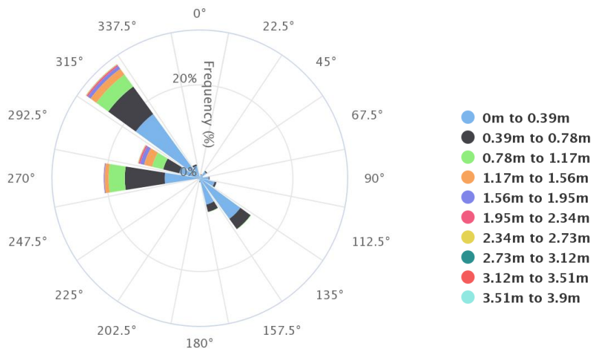
Figur 10 Vågros för signifikant våghöjd utanför Jonstorp (i Skälderviken) på ca. 15 m djup. Denna visar hur ofta (andel av tiden) vågorna kommer från en viss riktning. Våghöjden, i varje sektor, anges i en färgskala.
